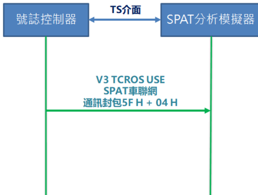
圖 3.1-1 TS1 測項互動圖
