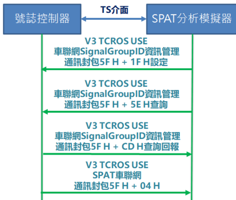
圖 3.3-1 TS3 測項互動圖
