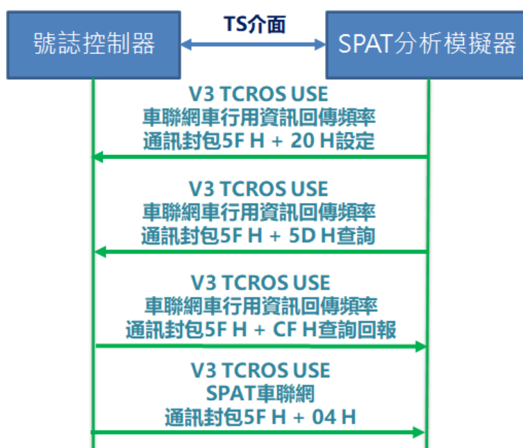
圖 3.4-1 TS4 測項互動圖
