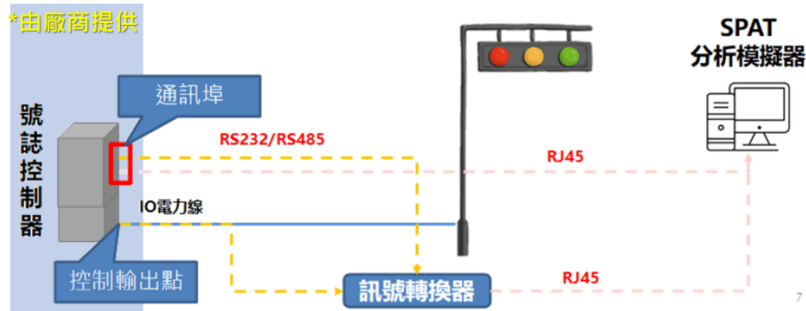
圖 2-1 號誌控制器與 SPAT 分析模擬器實體測試架構
