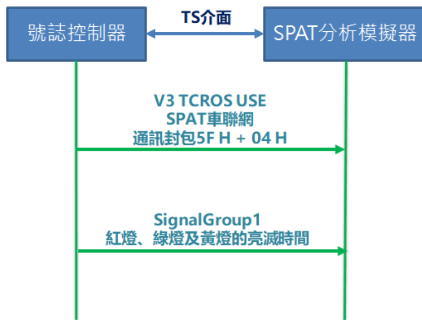
圖 3.2-1 TS2 測項互動圖
